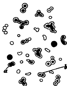
Fig. 15. 20-proc. Albumose, gefällt mit 7-proc. HgCl 2 ; Eisenhämatoxylin. Figurenerklärung siehe p. 34.
